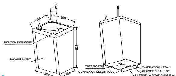
Plan d'installation
