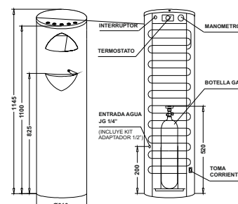
Plano de instalación
